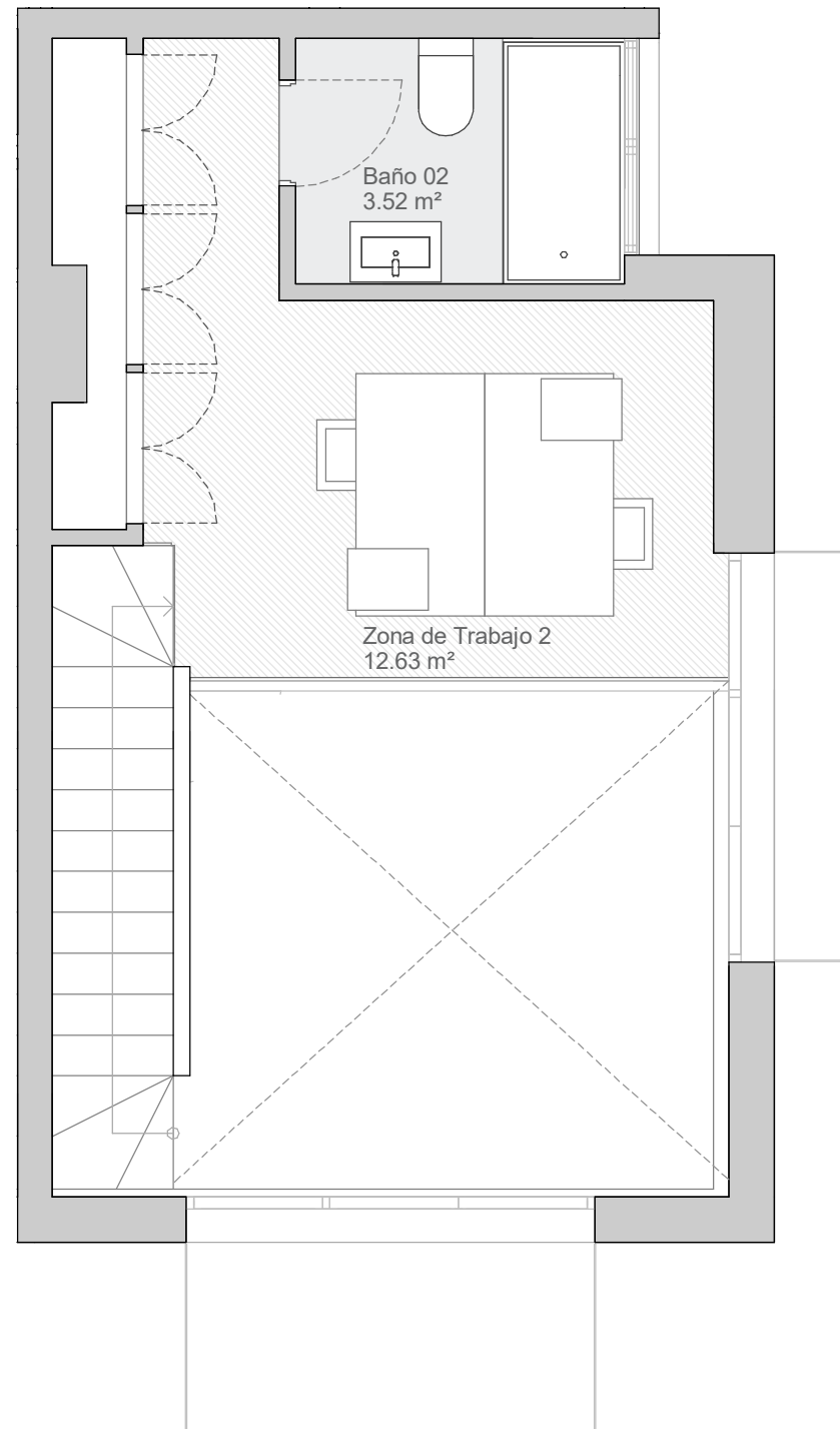
Planta entreplanta
