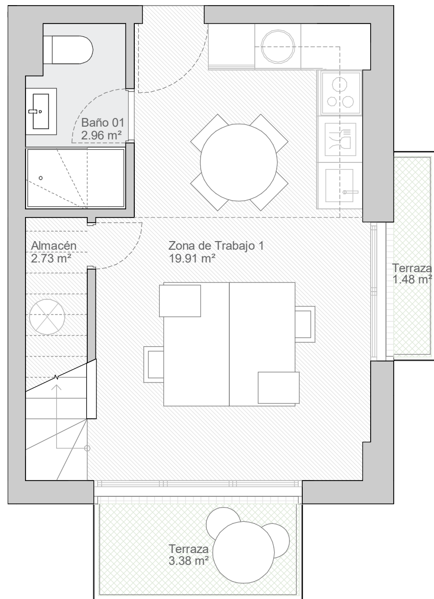
Planta segunda
